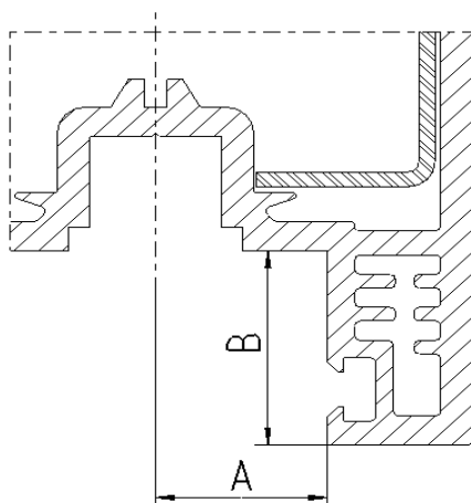
KŘÍDLO
